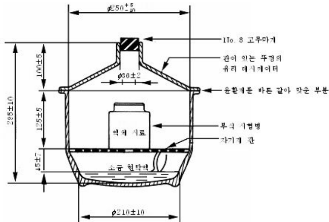
그림 3 습윤 장치
