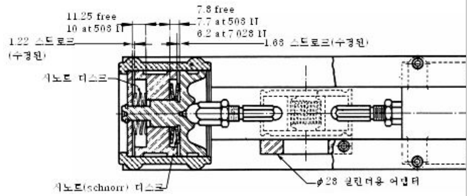
그림 4 스트로킹 시험장치
