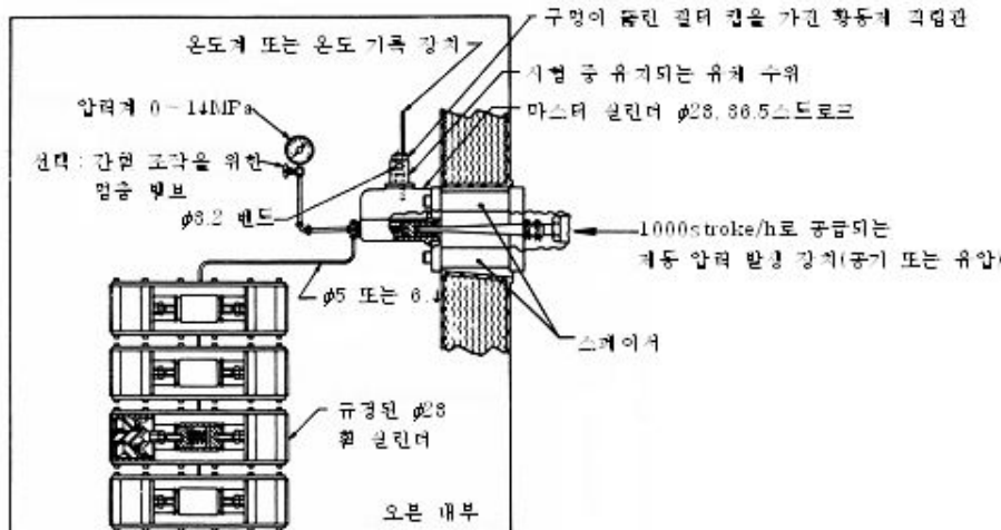
그림 4 스트로킹 시험장치
