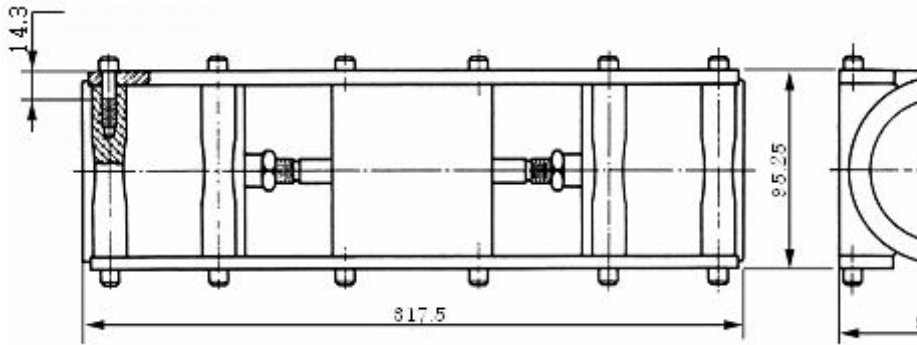
그림 5 그림 4의 상세도
