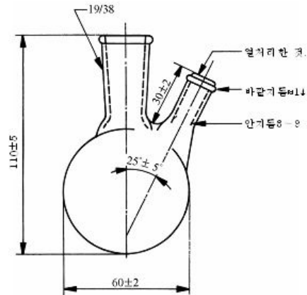
그림 2 100 mL 목이 짧은 플라스크의 상세도
