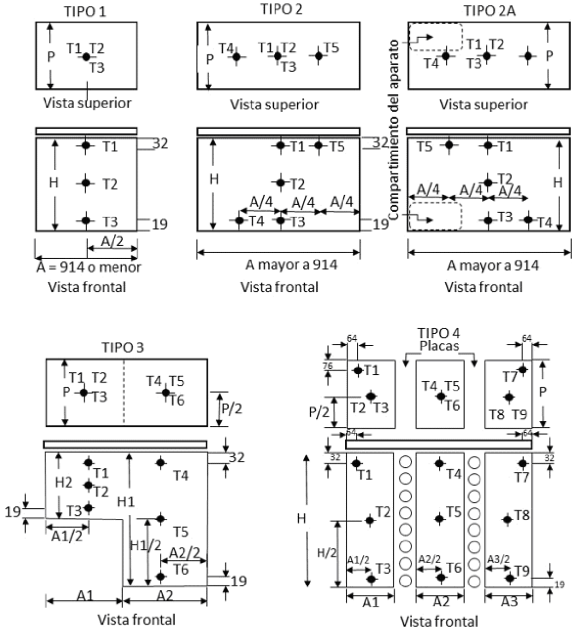
Figura A.4 Ubicación de los termopares para determinar la temperatura de los compartimentos congeladores de los refrigeradores y congeladores.
