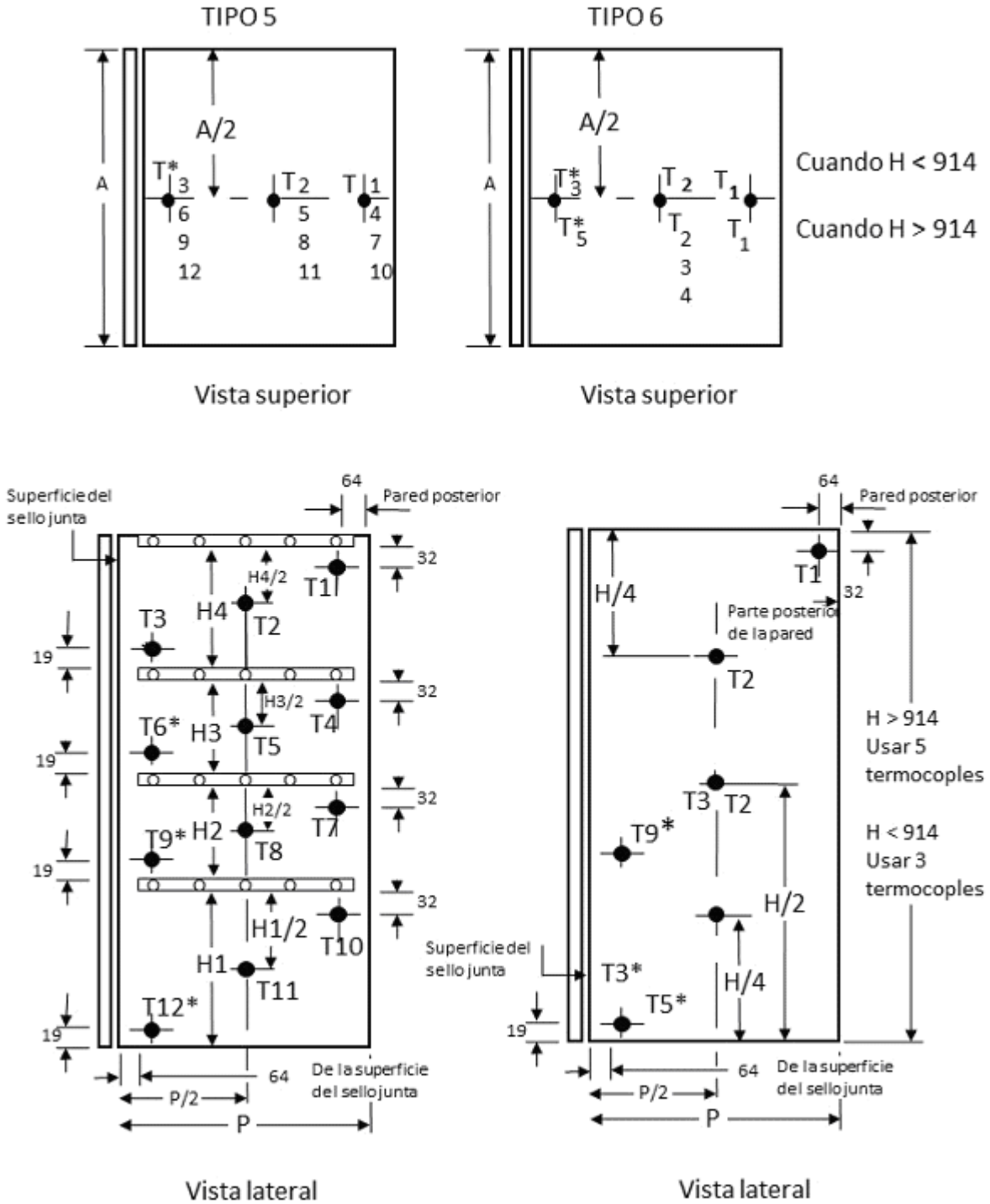
Figura A.4 (continuación) Ubicación de los termopares para determinar la temperatura de los compartimentos congeladores de los refrigeradores y congeladores.
