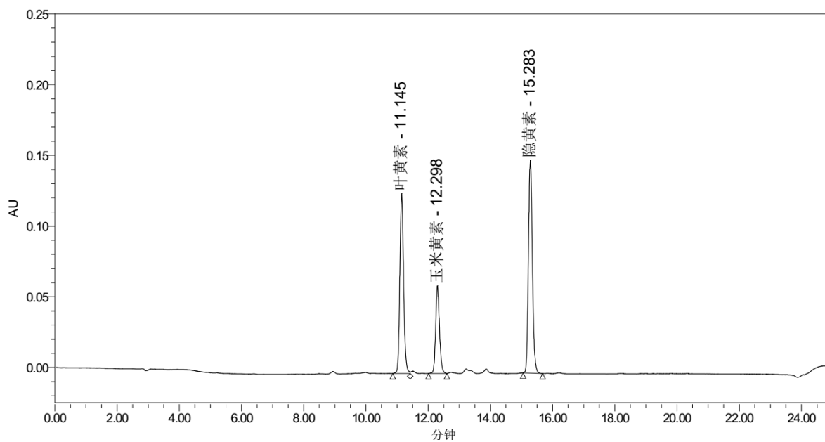
图 B.1 玉米黄素、隐黄素和叶黄素标准溶液的液相参考色谱图
