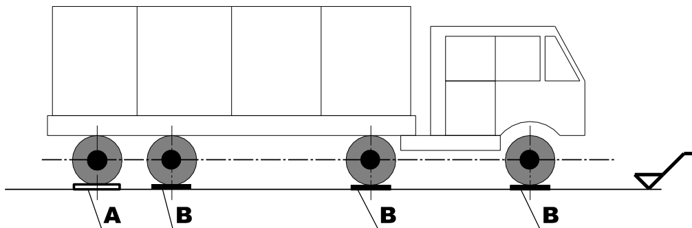
Obrázek 3 – Použití zařízení a vyrovnávacích desek
