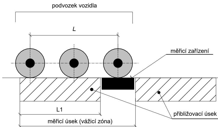
Obrázek 2 – Měřicí úsek zařízení
