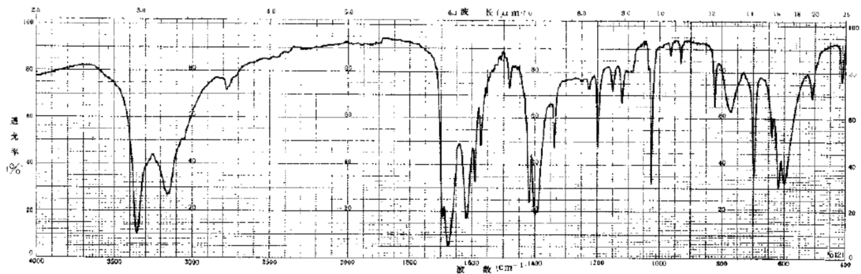
图B.1 烟酰胺标准品红外光谱吸收
