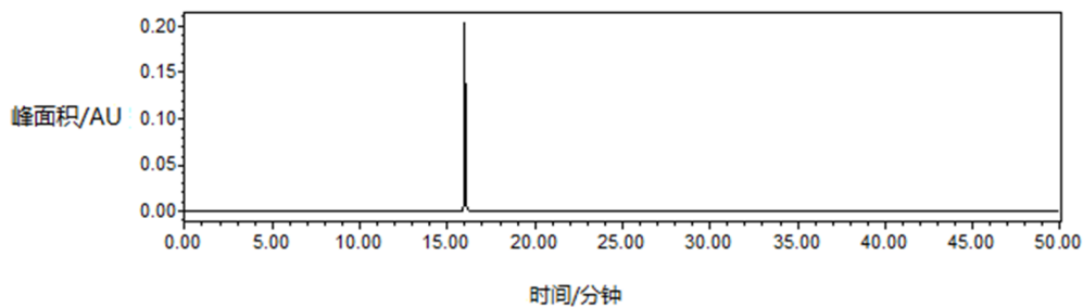
图B.2 羟钴胺试样品色谱图
