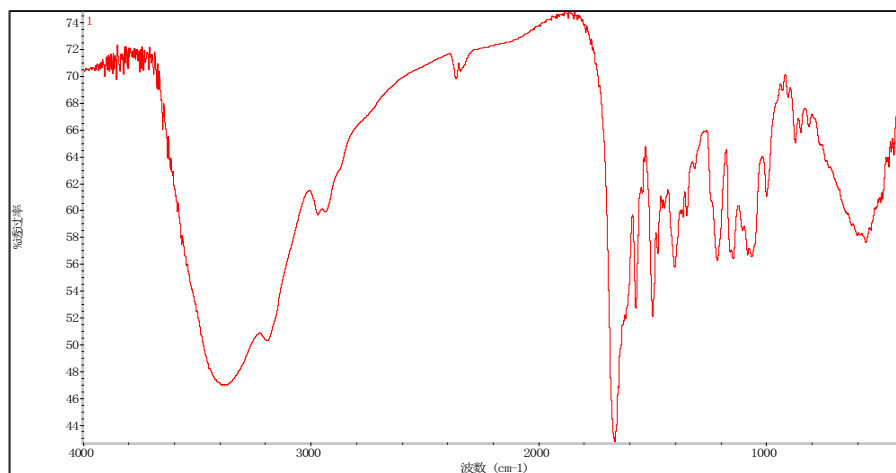
图B.1 盐酸羟钴胺标准红外光谱图
