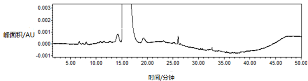
图B.3 羟钴胺试样有关物质色谱图
