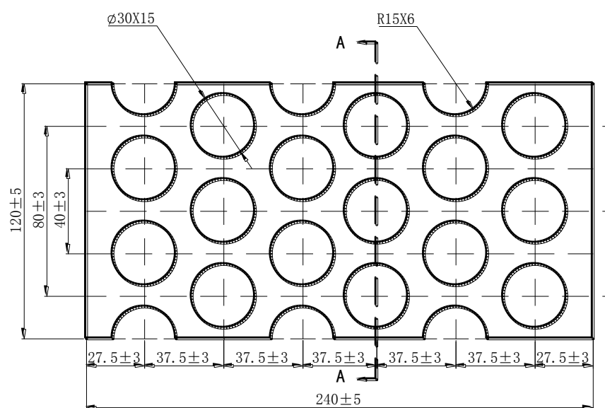
图 A.1 耐火砖尺寸
