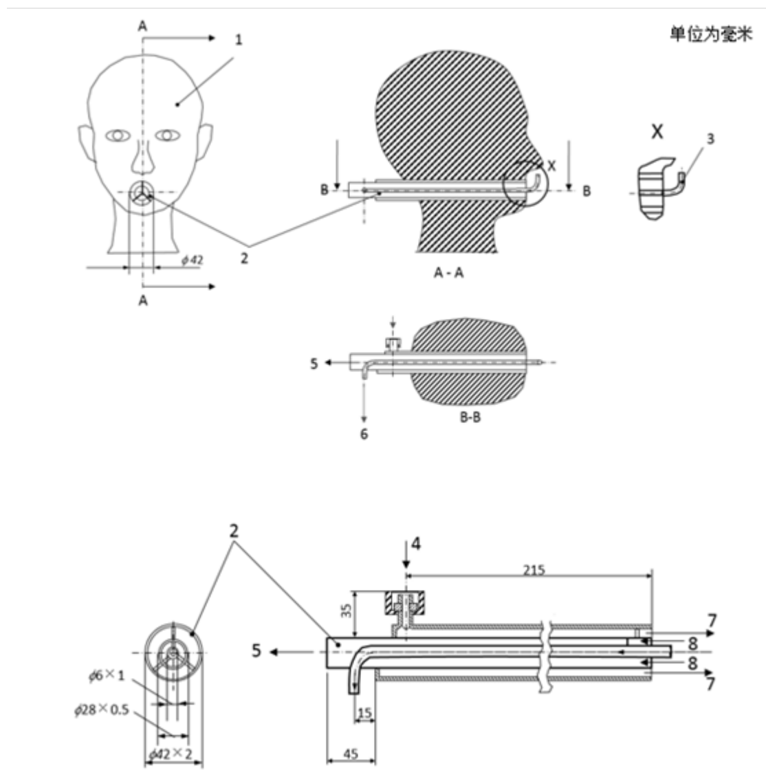
图3 呼气阻力和吸气阻力检测装置示意图
