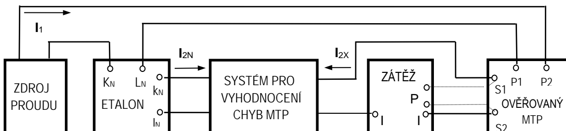
Obrázek 3 – Základní uspořádání pro určení chyb měřicího transformátoru proudu
