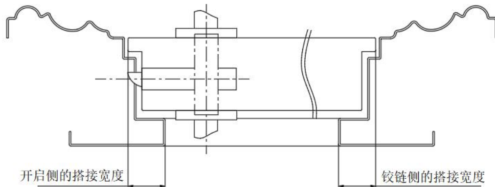
图 1 框扇搭接宽度示意图
