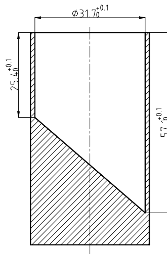
图 19 小零件圆筒
