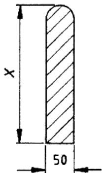
a) Round top edging: Type ER
