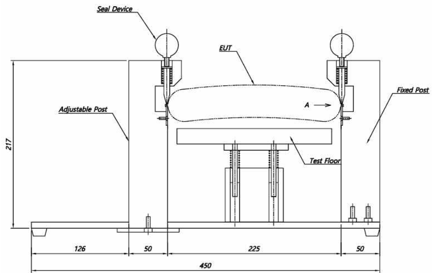
그림 101(b) 밀봉을 위한 지그
