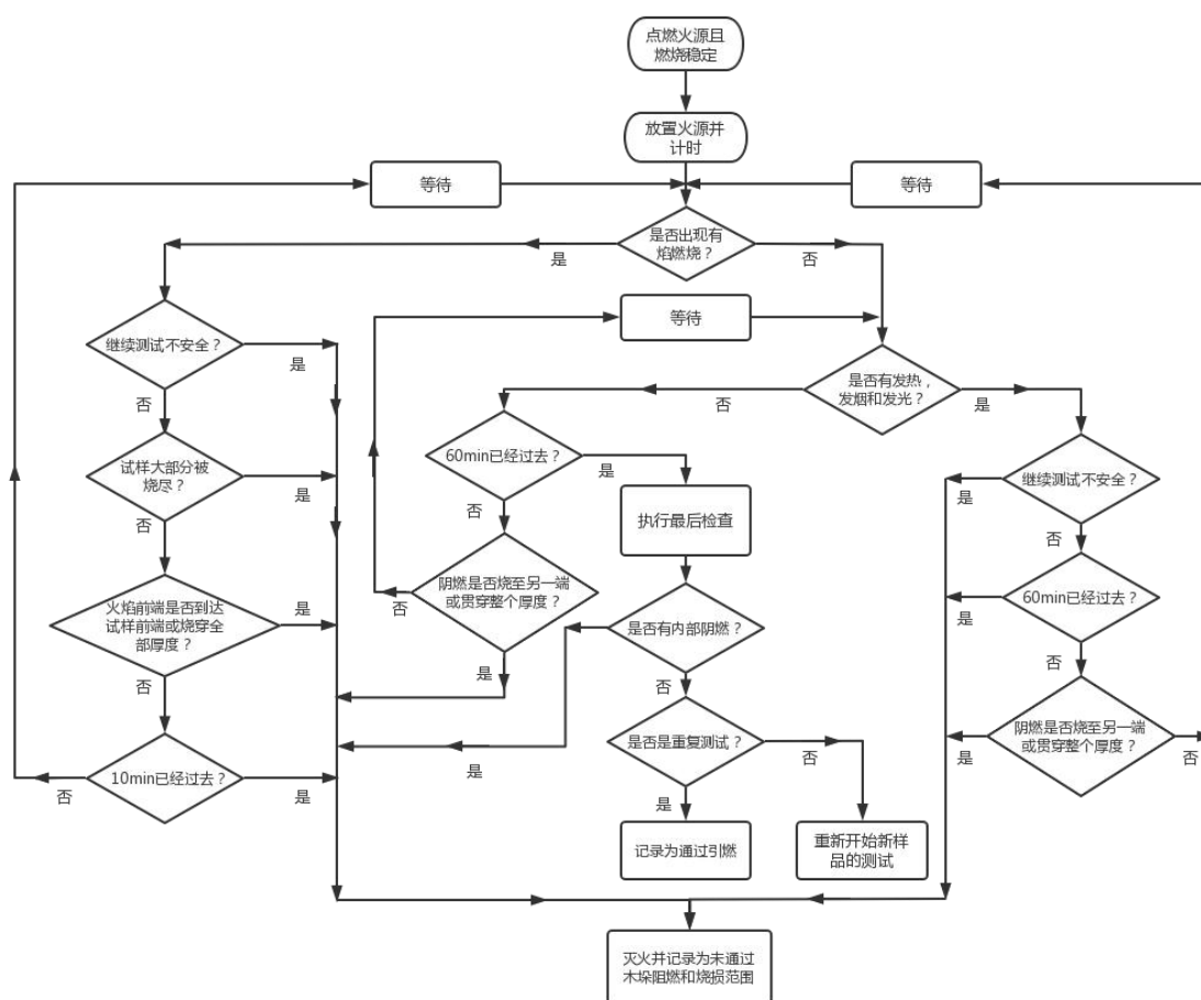
图 C.3 木垛试验流程图
