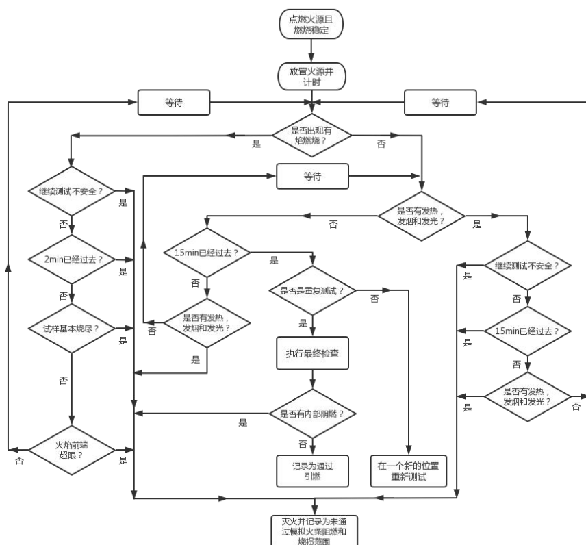
图 B. 1 模拟火柴火焰引燃流程图
