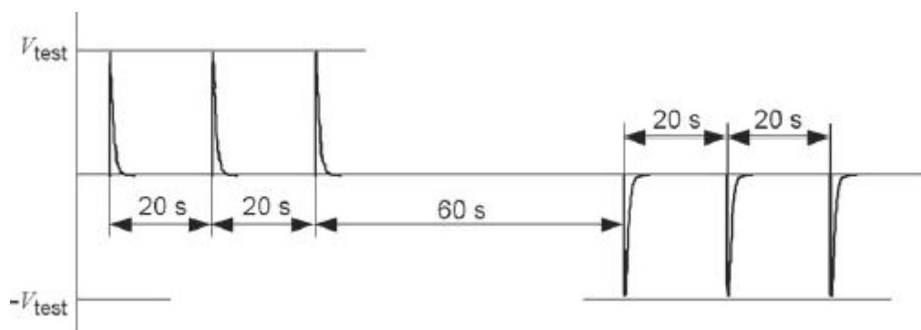
图3 试验1和试验2中的时序
