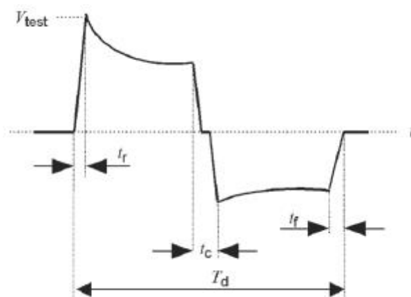
图 5 试验 2 双相除颤波形
