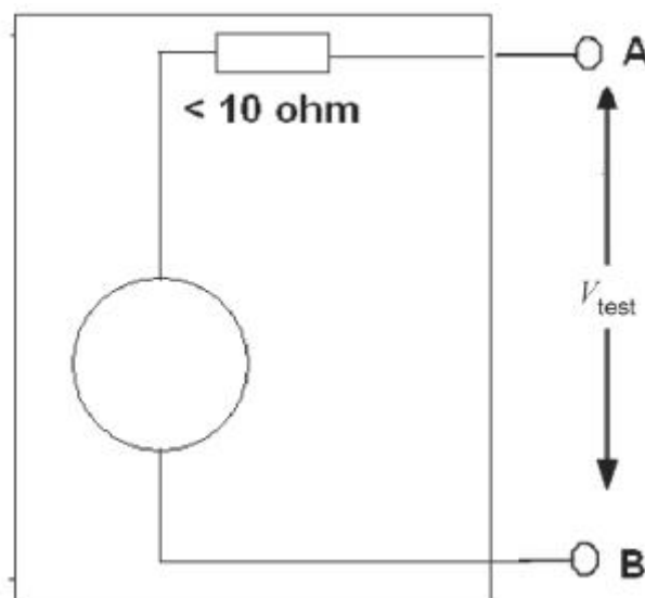
图2 除颤试验电压发生器
