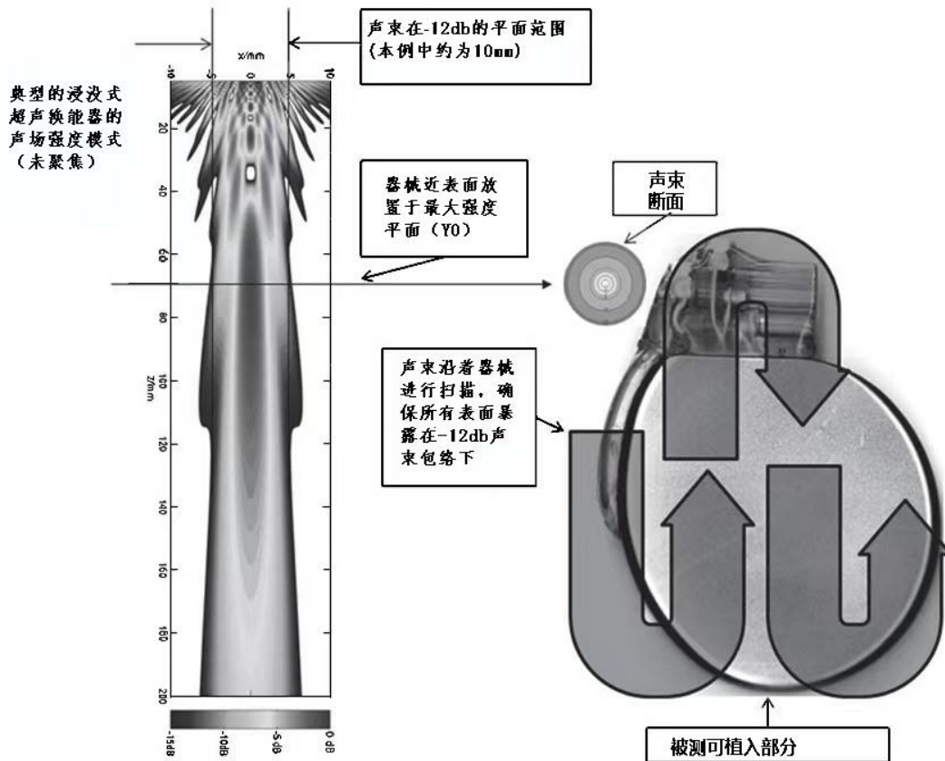
图 A.2 在植入部分上超声场暴露的定位和扫描
