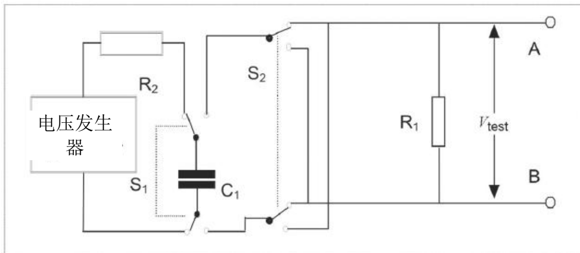
图 4 截断指数除颤波形的试验布置
