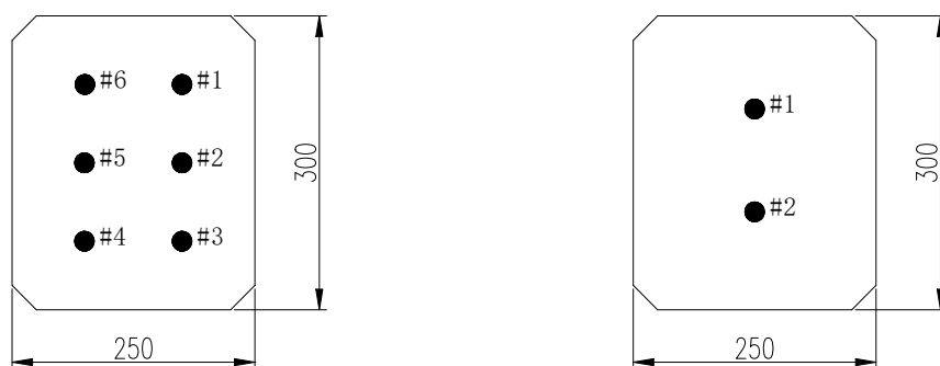
b) 防弹插板弹着点位置示意
