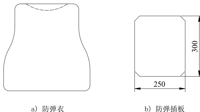
图 4 防弹层部件示意图
