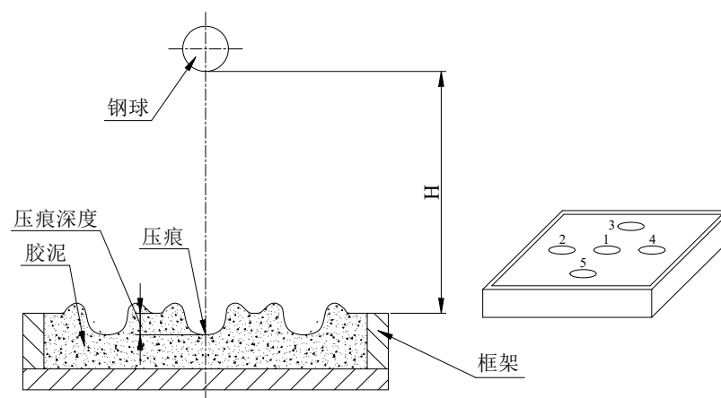
图 D.3 背衬材料冲击位置
