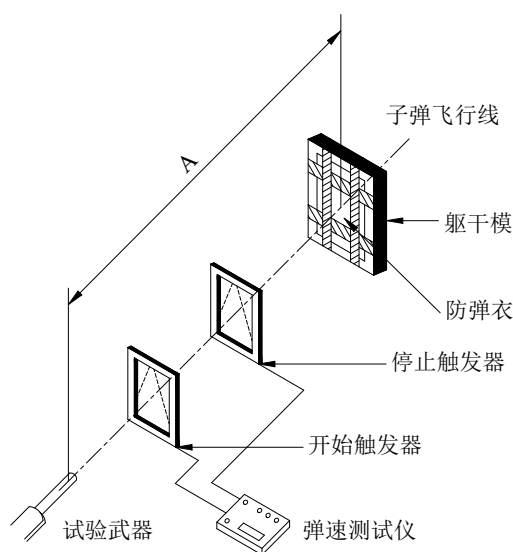
图 B.1 设备布置示意图
