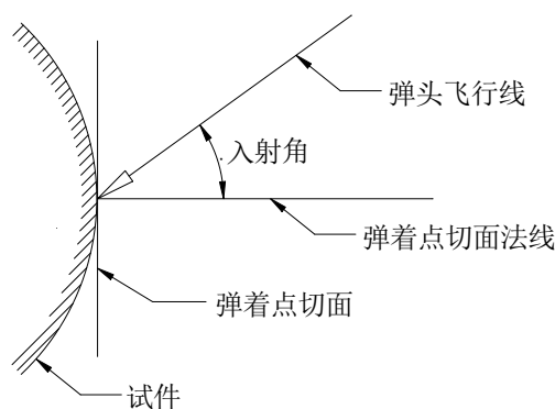
图1 入射角示意图
