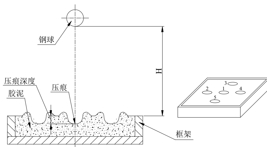
图 B.3 背衬材料冲击位置
