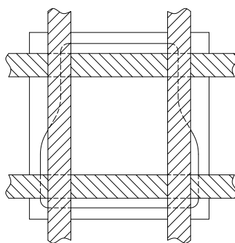
图 B.5 防弹衣试样固定
