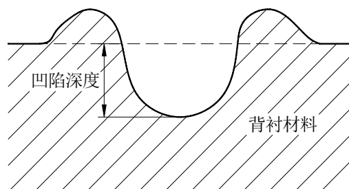
图 B.2 凹陷深度的测量
