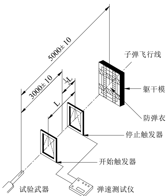
图 D.1 设备布置示意图
