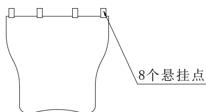
图 5 防弹层保护套悬挂示意图
