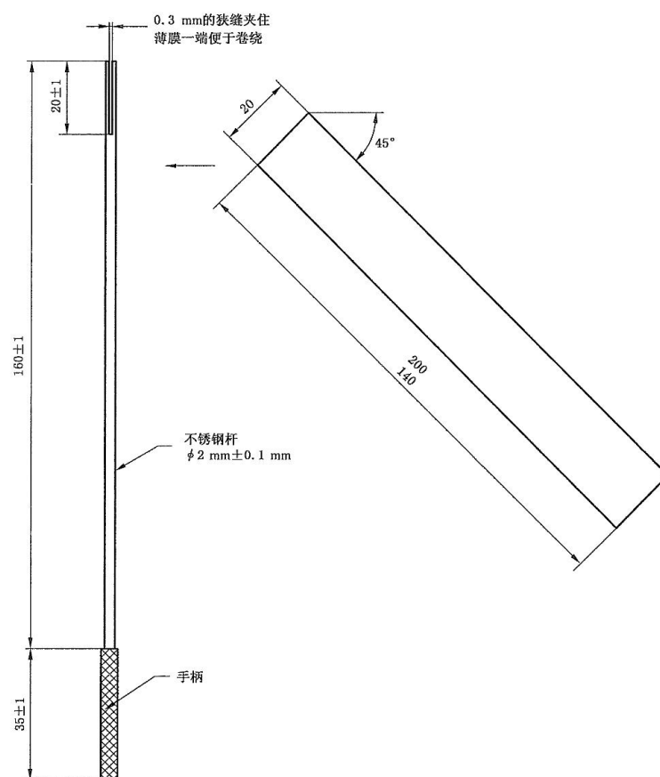
图 A. 3 非自撑试样的支撑框架
