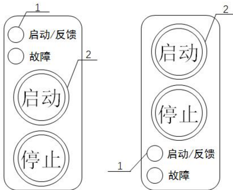
图3 控制开关横向布局
